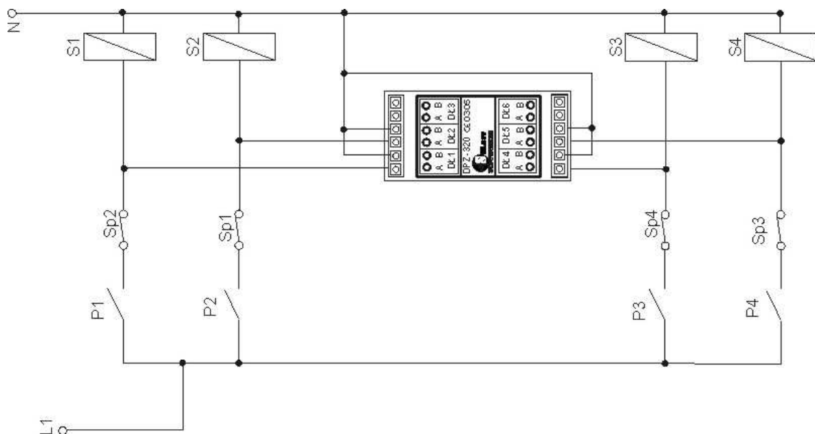
Podłączenie dławika DPZ-320 do cewek styczników
